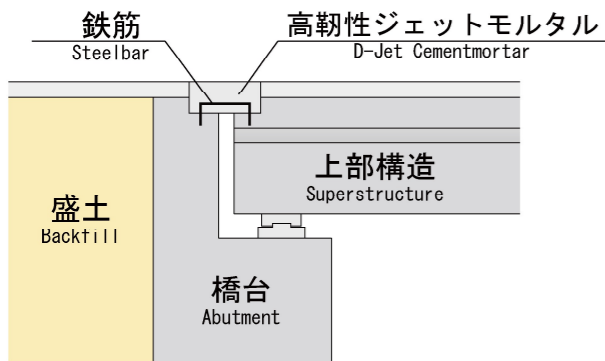
基本構造
