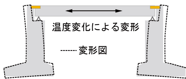
温度変化による橋体の挙動 ※1
