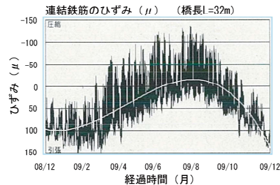
温度変化による連結鉄筋のひずみ ※1
