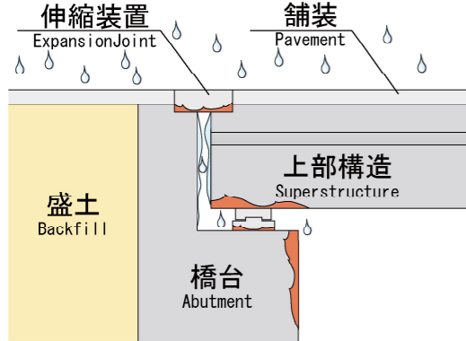
けた端部の劣化
