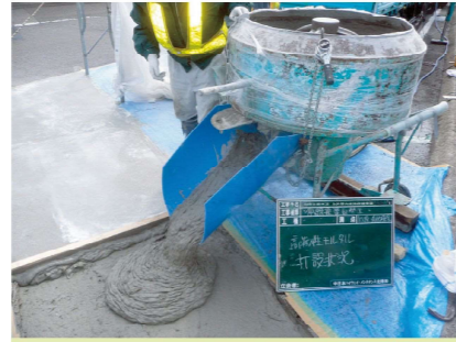
5. 高靱性ジェットモルタル打設
